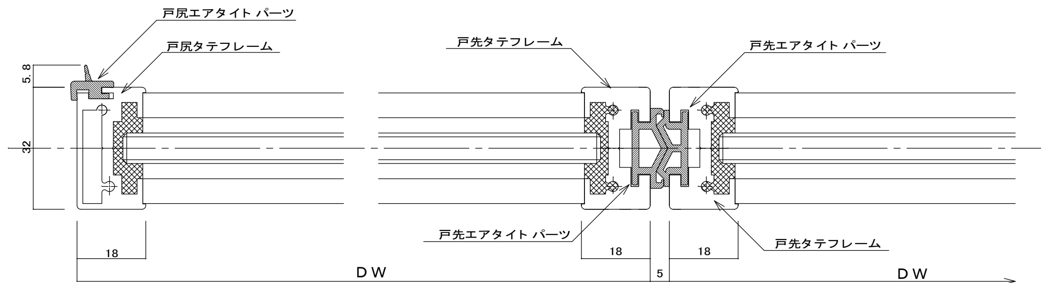
B-B 断面図 S=1/1
