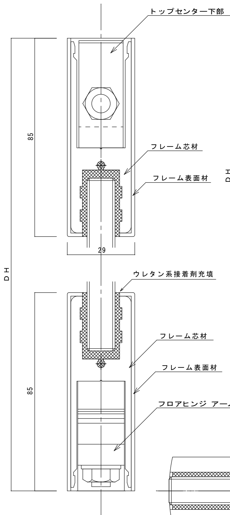
A-A断面図 S=1/1
